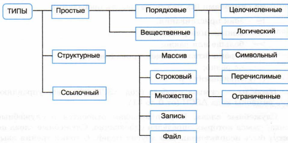
Рис. 3.10. Система типов данных Паскаля
